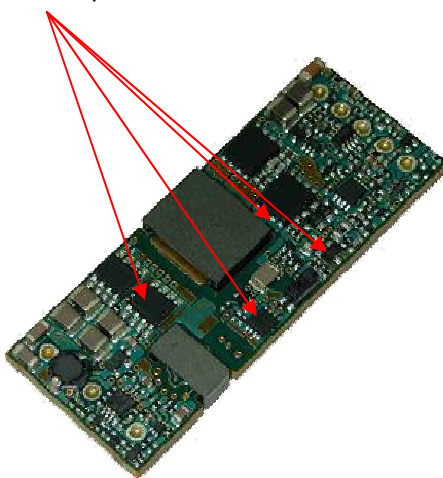
Thermocouples
